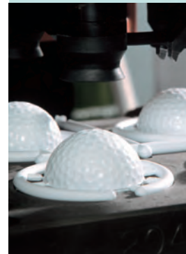
ボール成型 Ball molding
